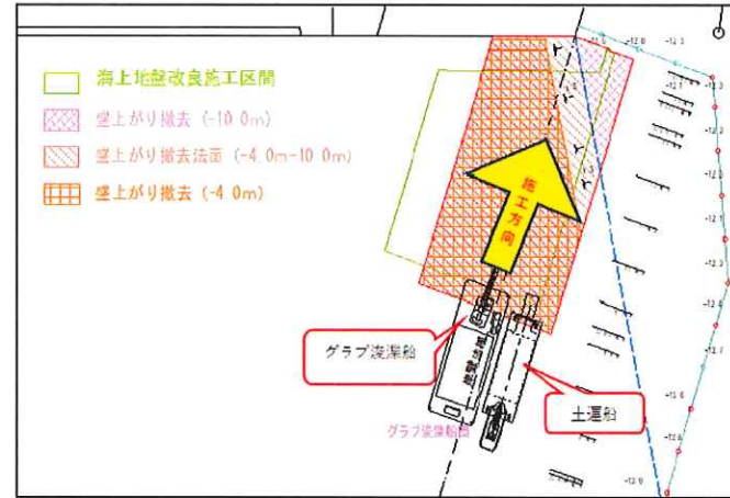
盛上り土撤去計画図
