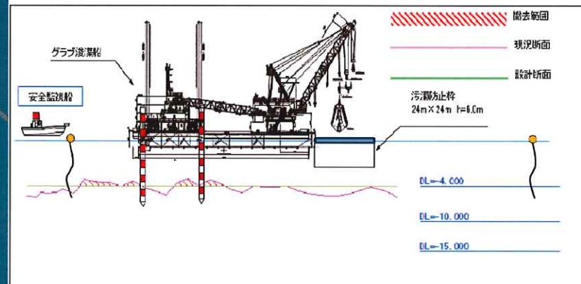
断面図
