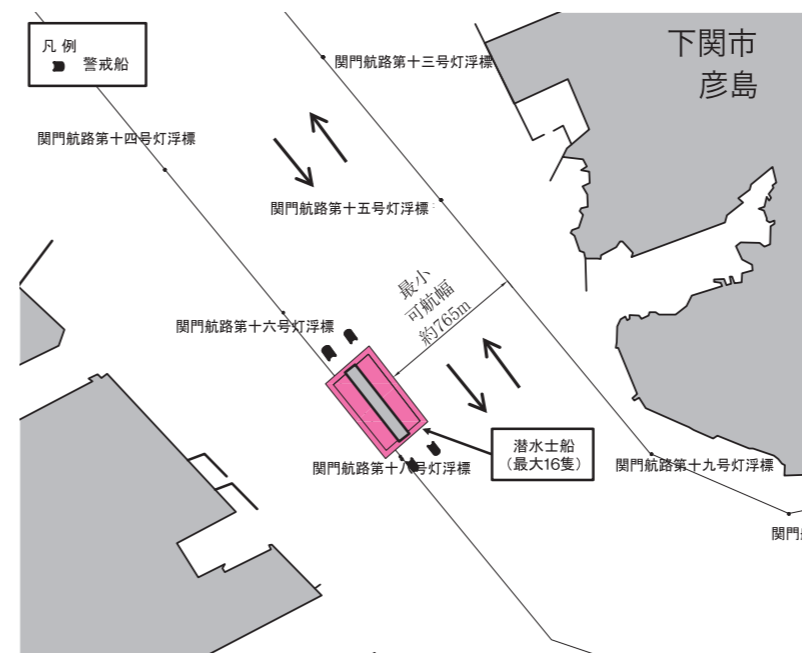
図-2 潜水士船・警戒船配置図【潜水探査時の例】 施工時の通航方法【F1・F2・F3工区】
