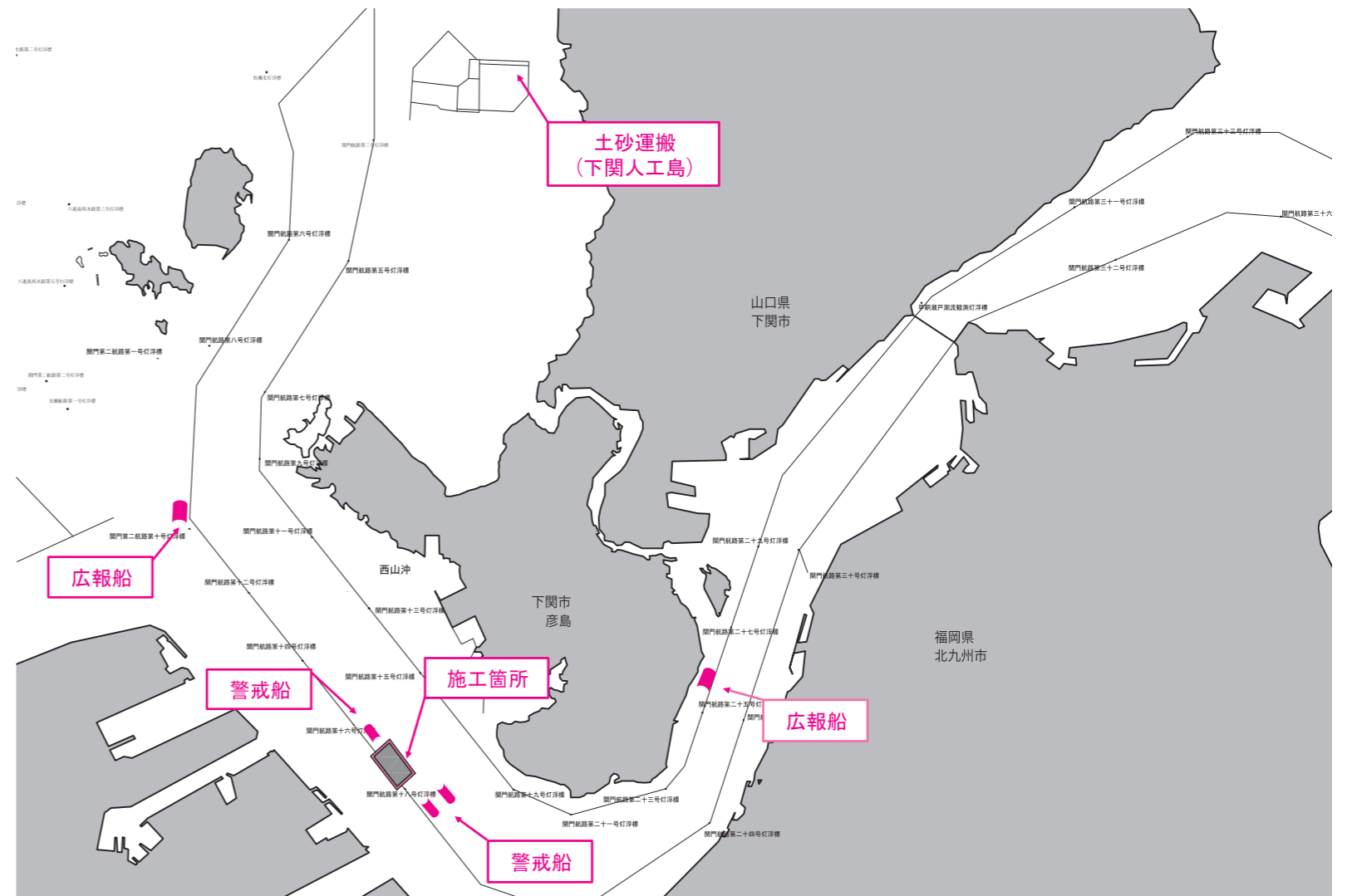
図-2 潜水士船・警戒船配置図【潜水探査時の例】 施工時の通航方法【F1・F2・F3工区】
