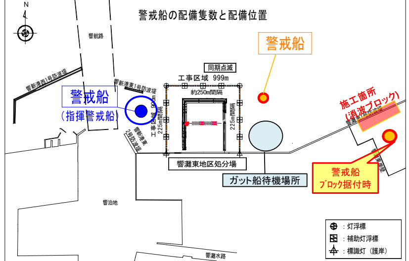
図-5 工事作業警戒船配置図
