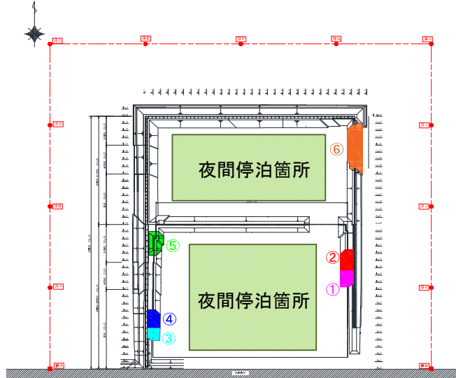
図-1 護岸築造工事位置図
