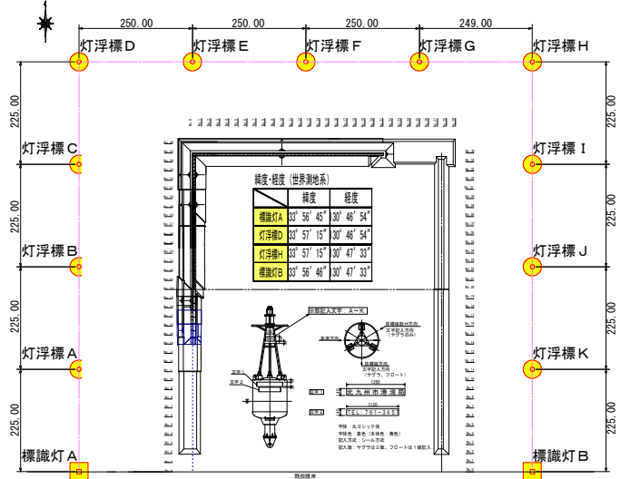
図-2 護岸築造工事平面図
