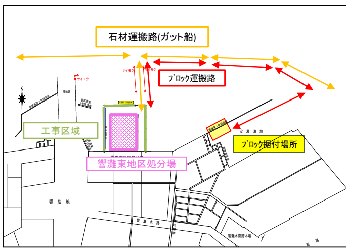
図-3 運搬経路図
