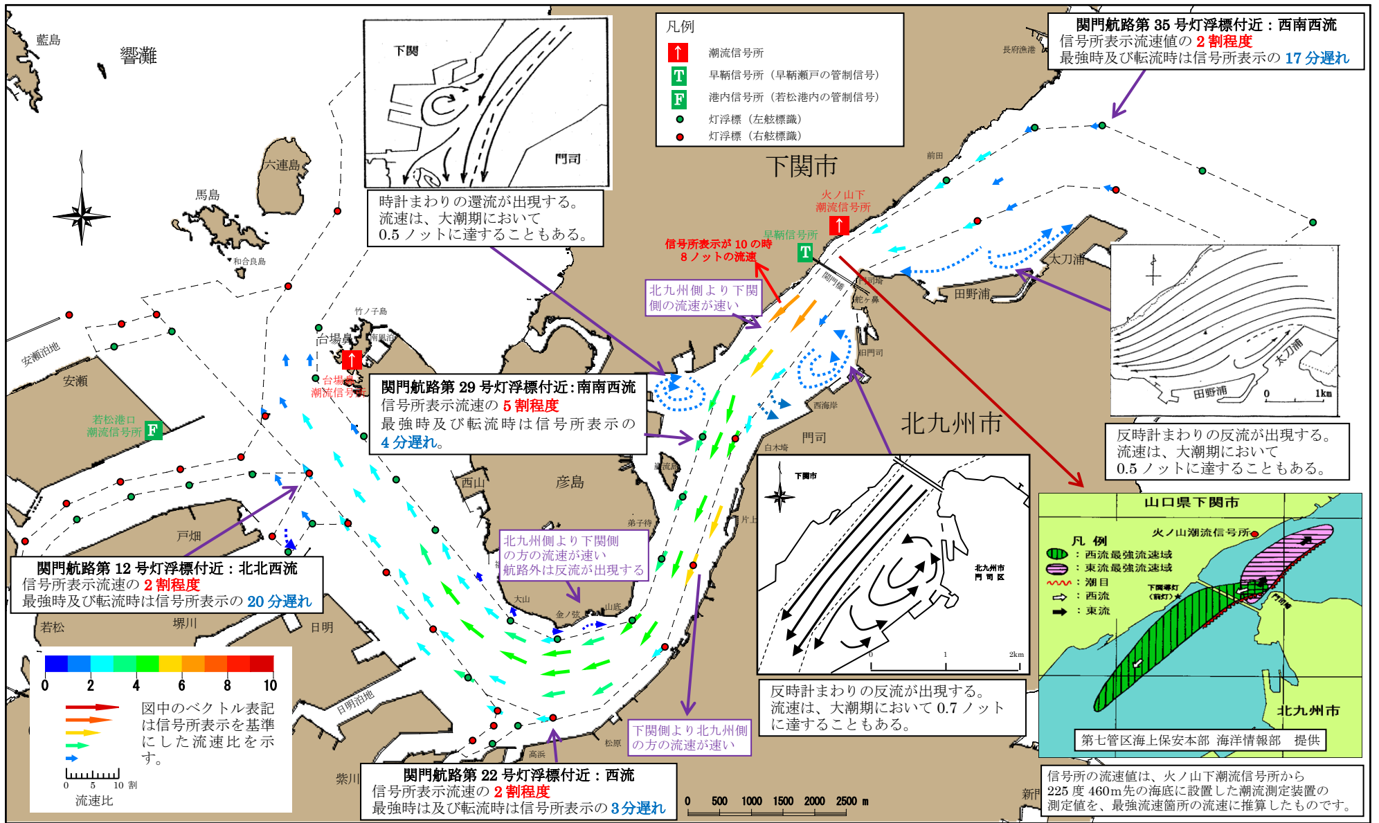
図2 関門航路潮流模式図 (西流時)：流速ベクトル色付け
