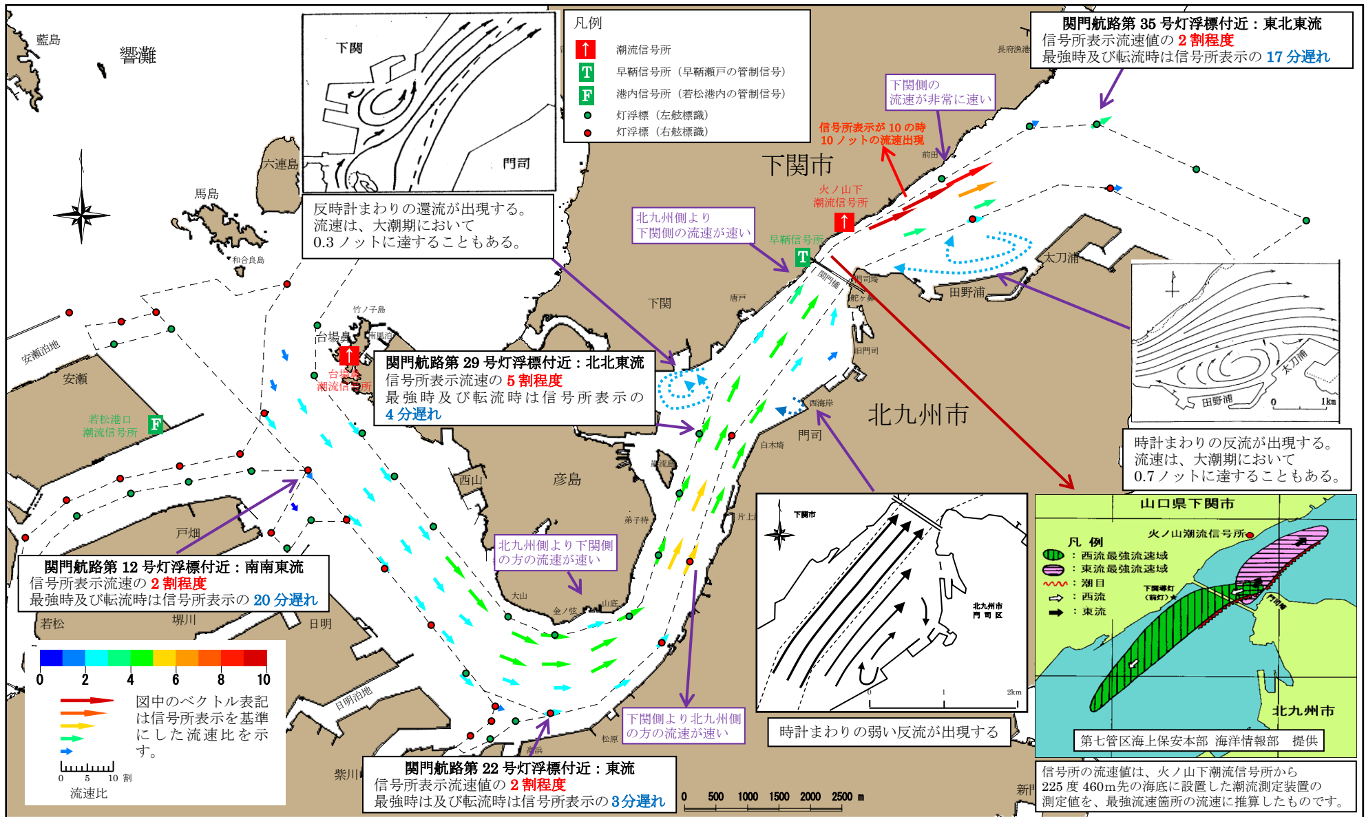
図 4 関門航路潮流模式図 (東流時) : 流速ベクトル色付け
