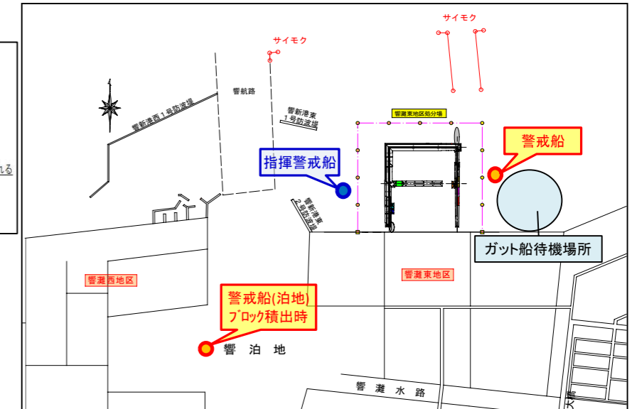
図-5 工事作業警戒船配置図
