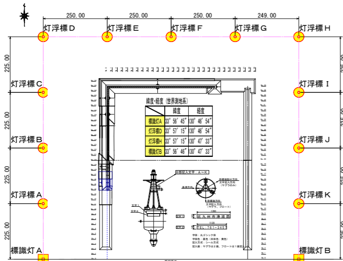
図-2 護岸築造工事平面図
