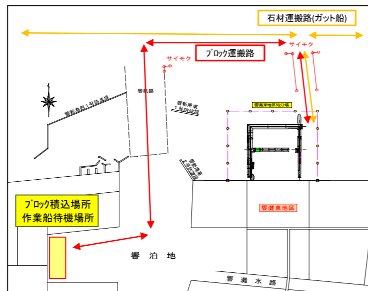
図-3 運搬経路図
